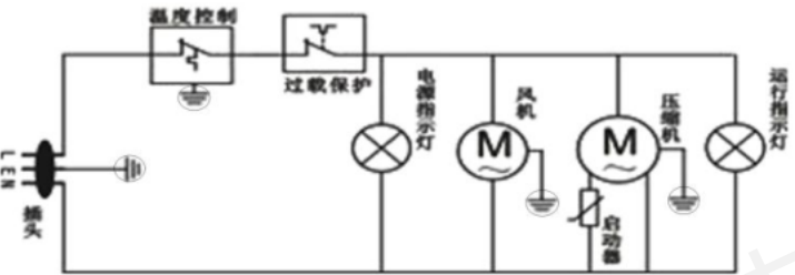
电气原理
