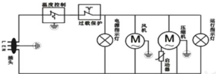
电气原理
