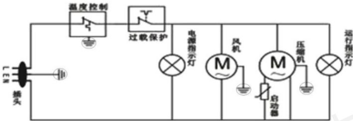
电气原理
