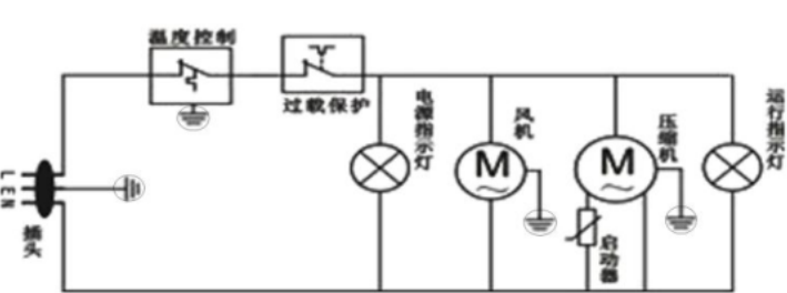
电气原理
